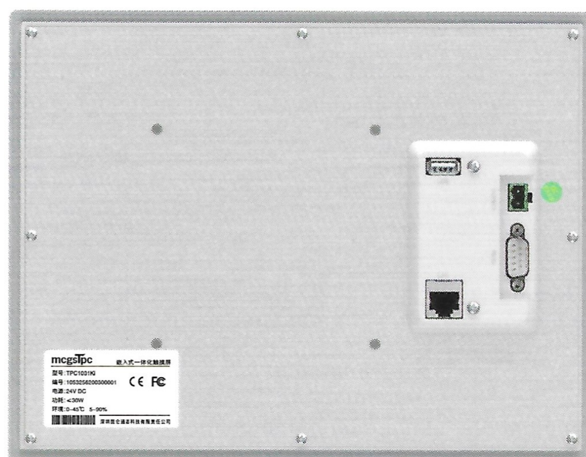
◎ Ki系列接口图
