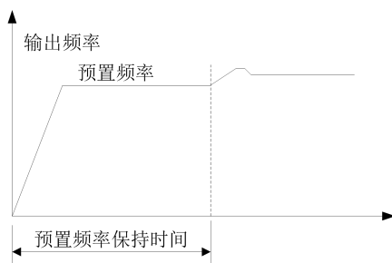
图 6-24 闭环预置频率运行示意图
