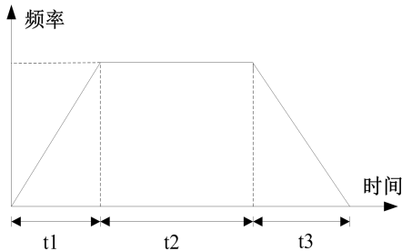
图 6-9 点动运行参数说明
