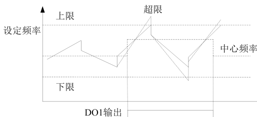
图 6-15 摆频运行上下限限制示意图
