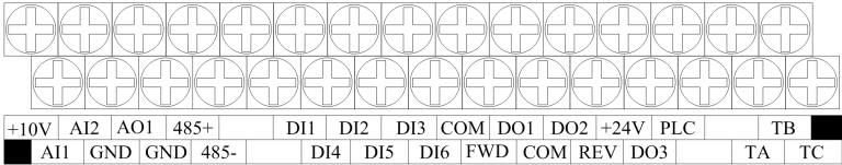
图 3-19 控制板端子排列顺序图 (0.7~7.5KW 控制板)
