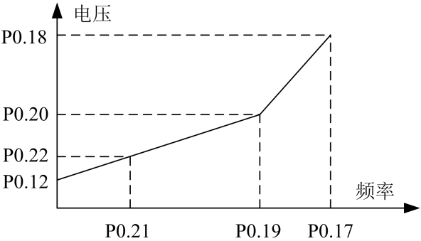
图 6-5 V/F 自定义曲线设定
