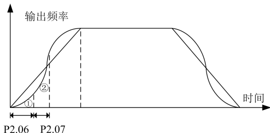
图 6-7 S 加减速曲线
