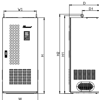
(d): 93KW~200KW 规格尺寸(壁挂)
