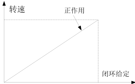
图 6-22 正特性示意图
