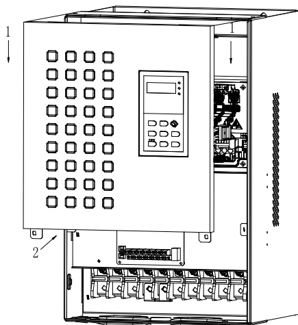
图 3-10 盖板的安装
