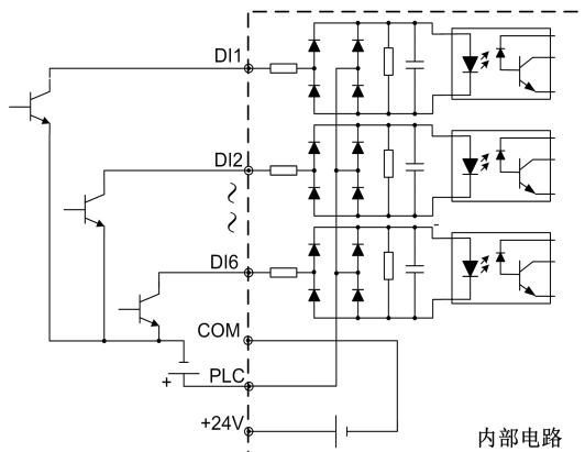
图 3-28 外部电源供电 NPN 图 (OC)
