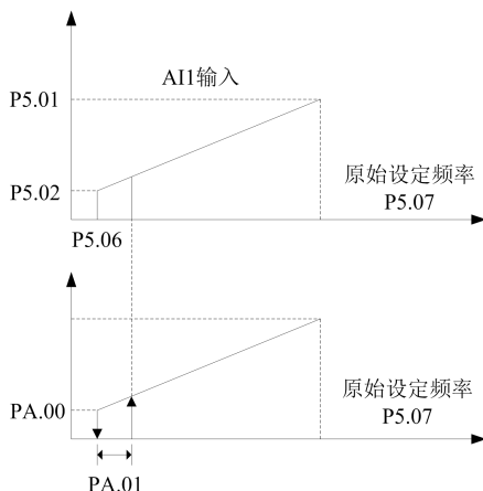
图 6-32 零频回差运行
