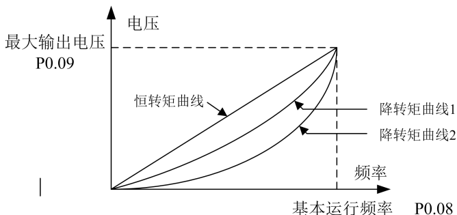
图 6-4 V/F 曲线
