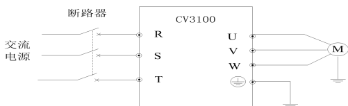
图 3-11 主回路简单配线
