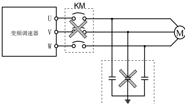
图 1-2 变频器输出端禁止使用电容器
