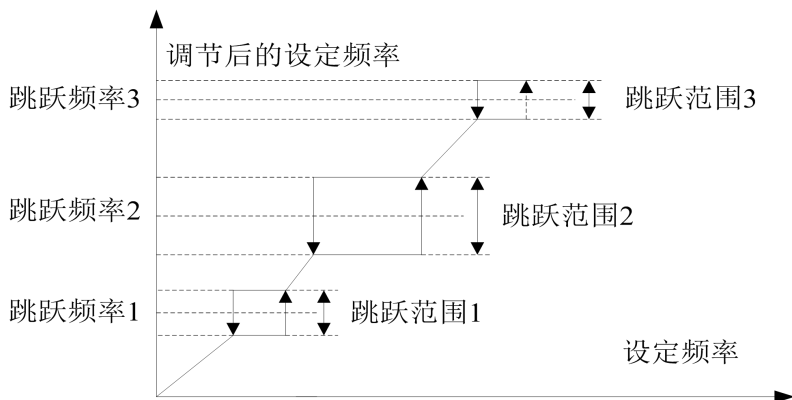
图 6-10 跳跃频率设定
