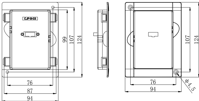
图 2-1 CV3100-LKD 外引托板尺寸（选配件）
