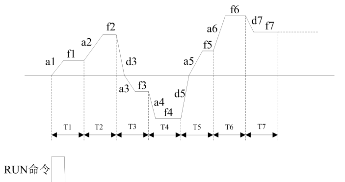
图 6-28 单循环后保持最终值示意图
