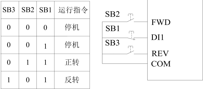
图 6-13 三线式控制模式 1
