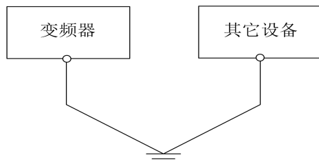
图 3-14 共用接地极示意图
