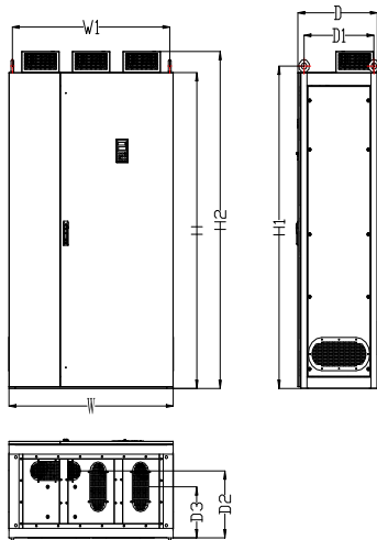
(j): 850KW 规格尺寸(柜机)
