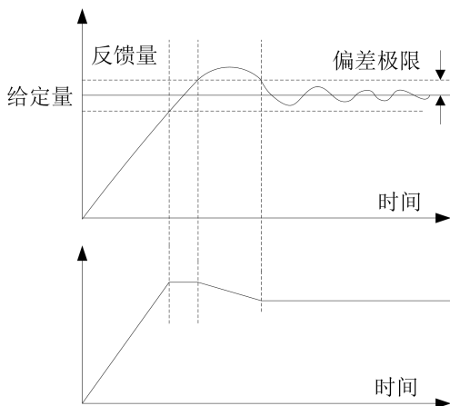
图 6-23 偏差极限示意图
