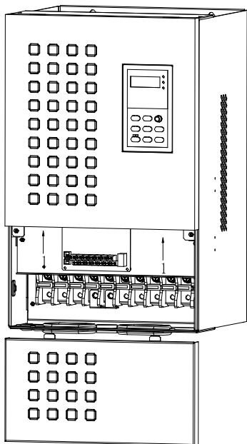
图 3-8 盖板的安装
