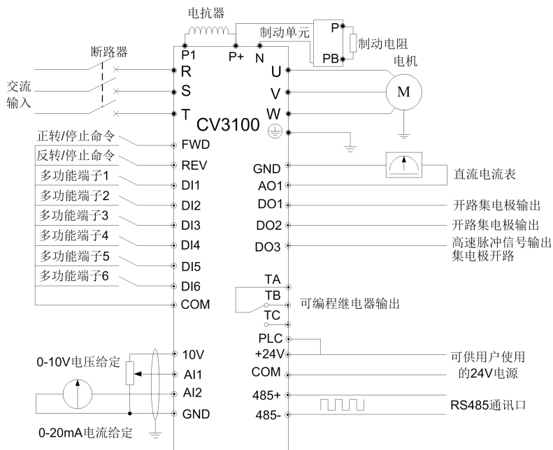
图 3-18 基本运行配线图
