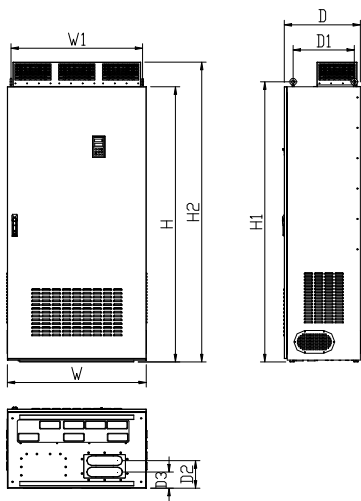
(i): 500KW~630KW 规格尺寸(柜机)
