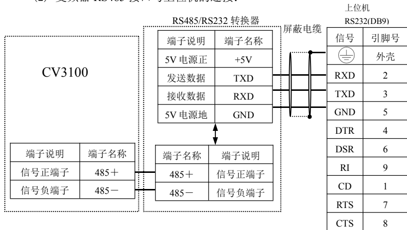
图 3-24 RS485—(RS485/232)—RS232 通讯配线
