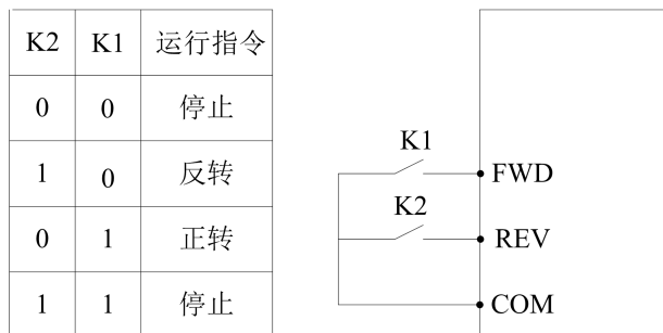
图 6-11 两线式控制模式 1
