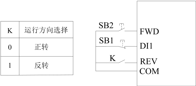
图 6-14 三线式控制模式 2
