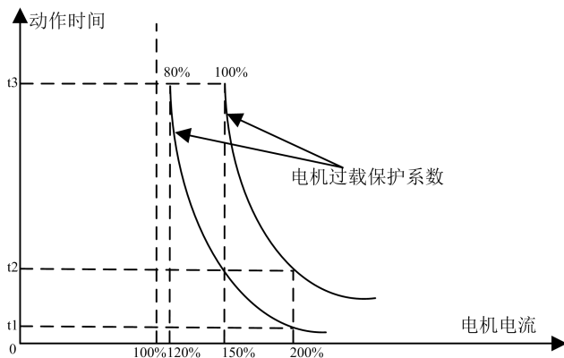
图 6-30 电机过载保护曲线示意图
