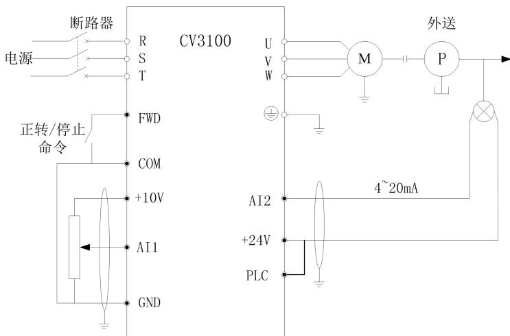
图 6-20 模拟反馈控制系统示意图
