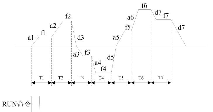
图 6-26 单循环示意图
