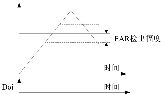
图 6-17 FAR 设定说明
