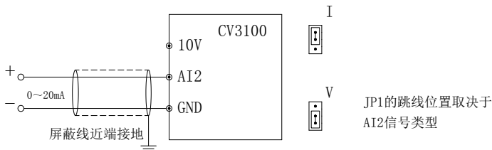
图 3-22 AI2 端子配线图
