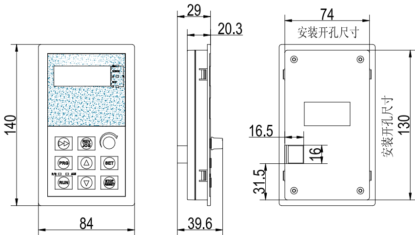
图 2-2 CV3100-RKD 键盘尺寸规格
