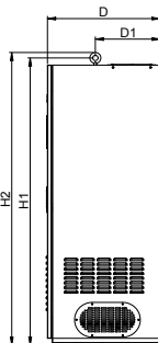
(d): 93KW~200KW 规格尺寸(壁挂)
