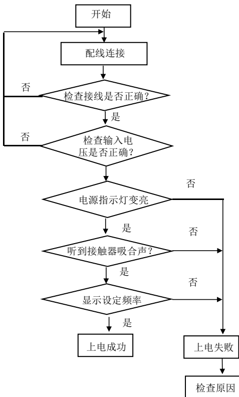
图 4-4 变频器初次上电操作流程
