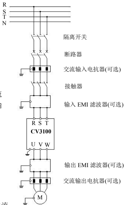
图 3-12 变频器与选配件的连接
