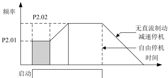
图 6-6 起动与停机频率输出曲线
