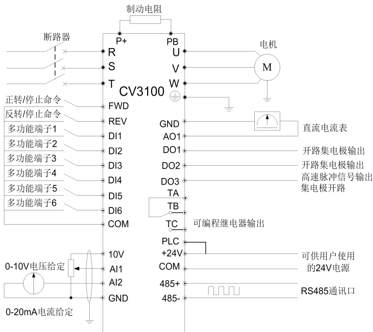
图 3-17 基本运行配线图
