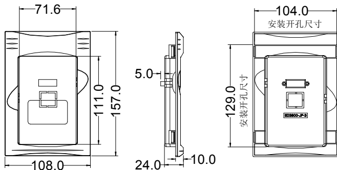
图 2-3 CV3100-RKB 托板尺寸 (RKB 键盘选配件)
