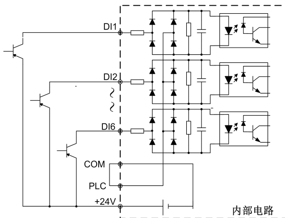
图 3-29 内部电源供电 PNP 图 (OE)
