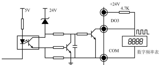
DO3 端口使用变频器内部 24V 电源的外部接线示意图
