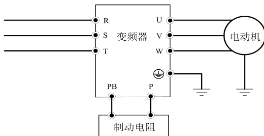
图 2-4 变频器与制动组件连线图（380V 18.5KW 以下）
