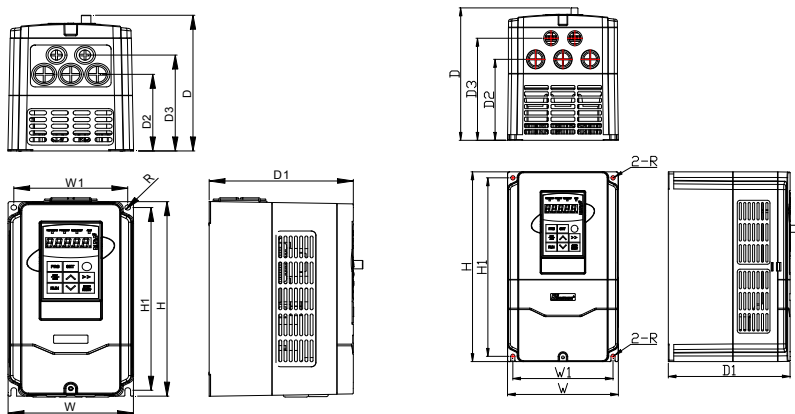
(a): 0.75KW~4.0KW 规格尺寸
