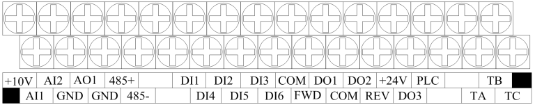
图 3-20 控制板端子排列顺序图 (11KW 以上控制板)
