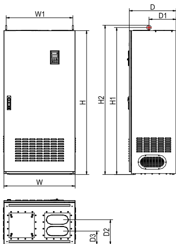
(g): 220KW~280KW 规格尺寸(柜机)
