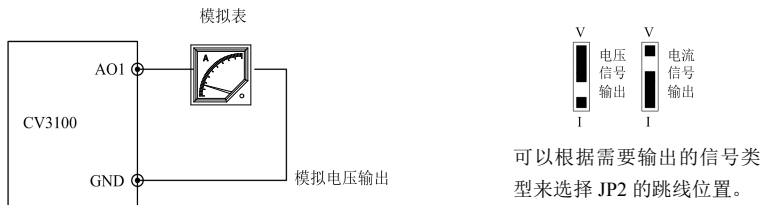
图 3-23 模拟输出端子配线
