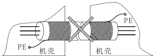
图 3-28 错误的屏蔽接地方法
