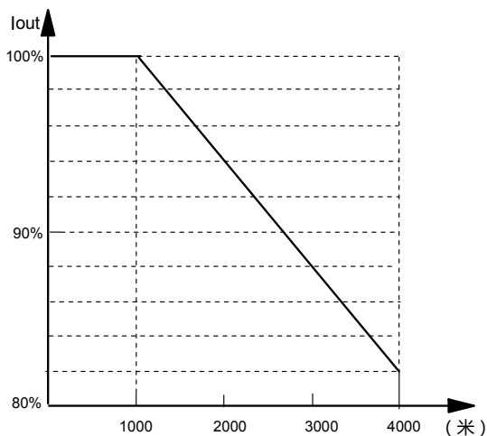
图 1-3 变频器额定输出电流与海拔高度降额使用图
