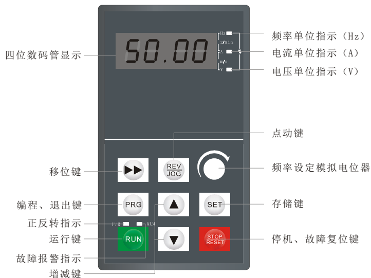
图 4-4 RKD 操作键盘示意图
