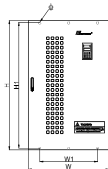
(c): 11KW~75KW 规格尺寸
