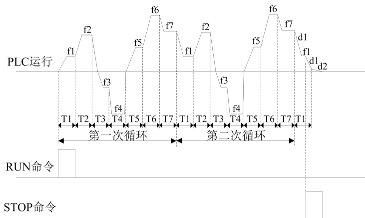
图 6-27 连续循环示意图
