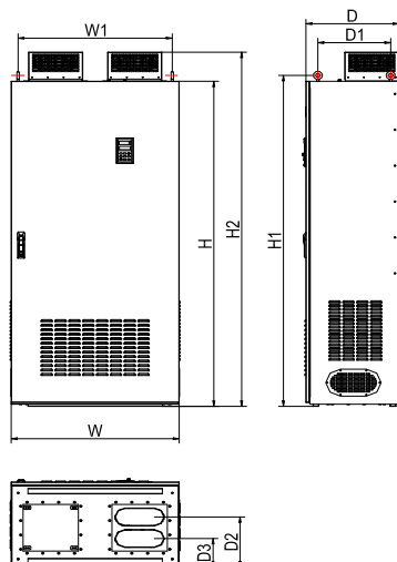
(h): 315KW~450KW 规格尺寸(柜机)
