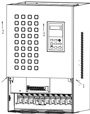
图 3-9 盖板的拆卸
