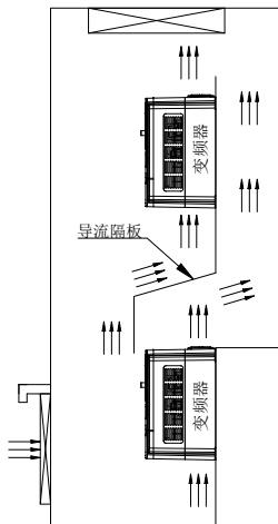
图 3-2 多台变频器的安装示意图
