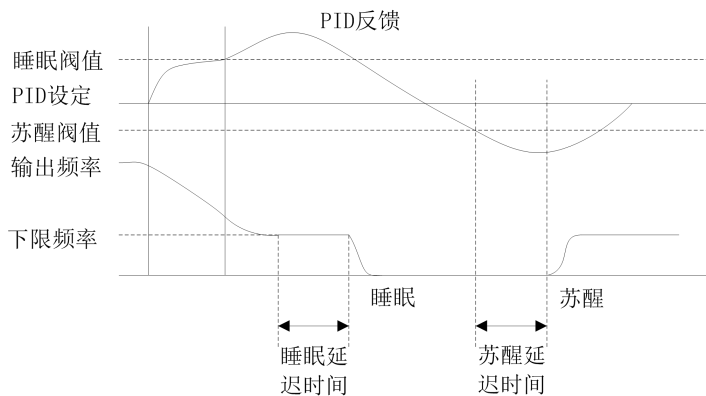
图 6-25 睡眠与苏醒功能示意图
