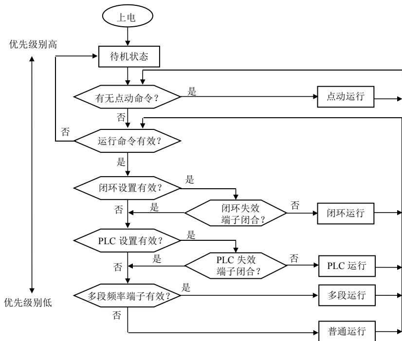
图 4-1 CV3100 变频器运行状态的逻辑关系图
