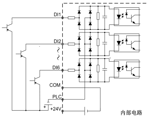
图 3-30 外部电源供电 PNP 图 (OE)
