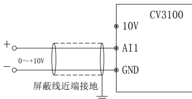
图 3-21 AI1 端子配线图
