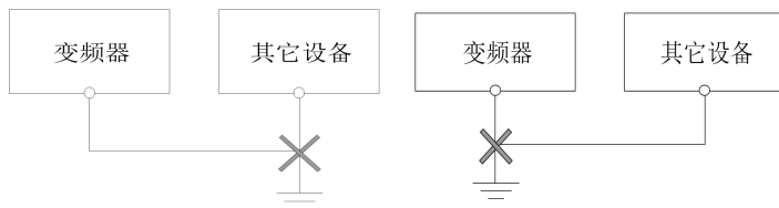
图 3-15 共用接地极示意图 (a)
