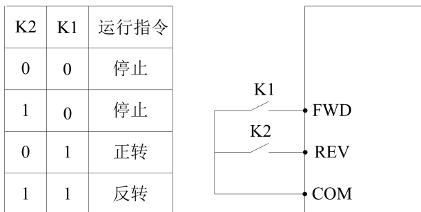
图 6-12 两线式控制模式 2
