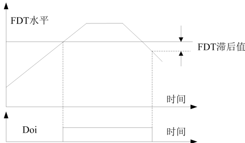
图 6-16 FDT 设定说明
