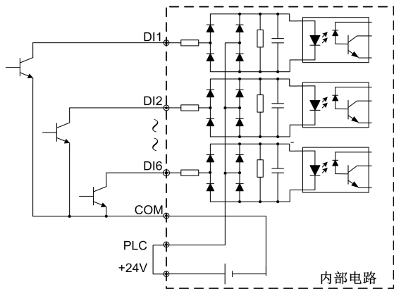
图 3-27 内部电源供电 NPN 图 (OC)
