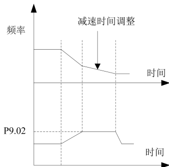
图 6-31 过压限制水平说明
