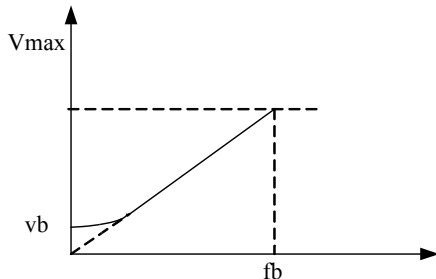
图 6-1 转矩提升设置
