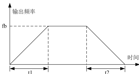
图 6-3 加速时间和减速时间设置说明
